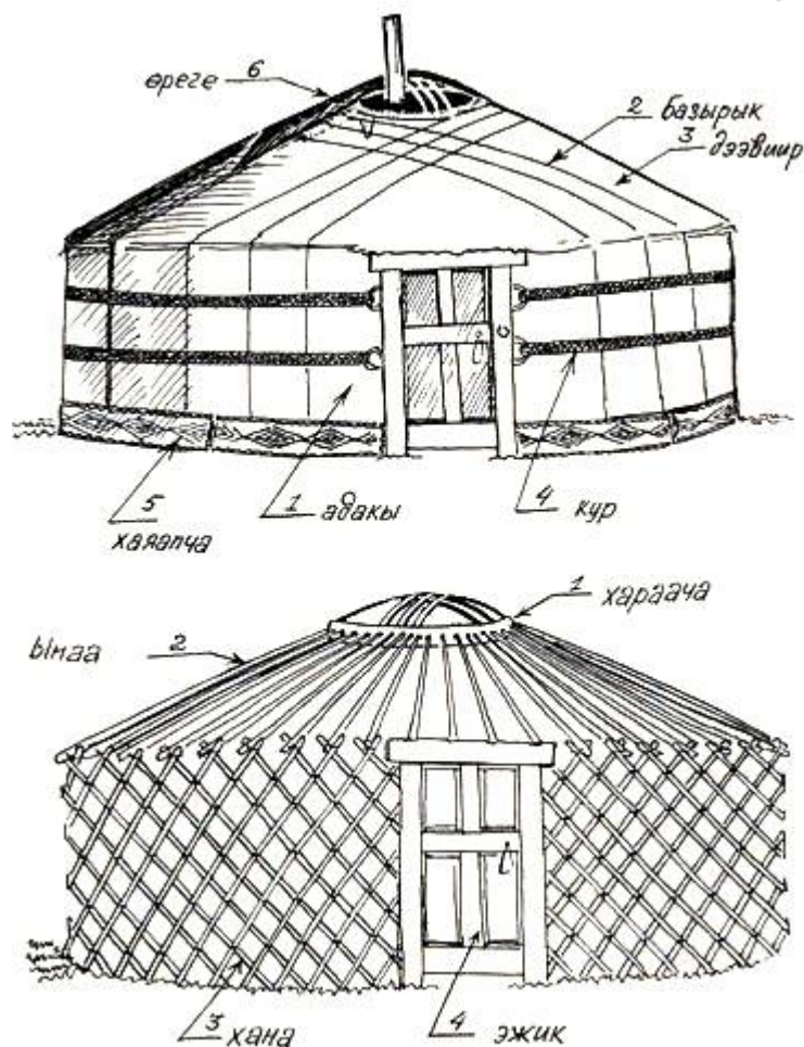
Рис. 2. Конструкция юрты.
